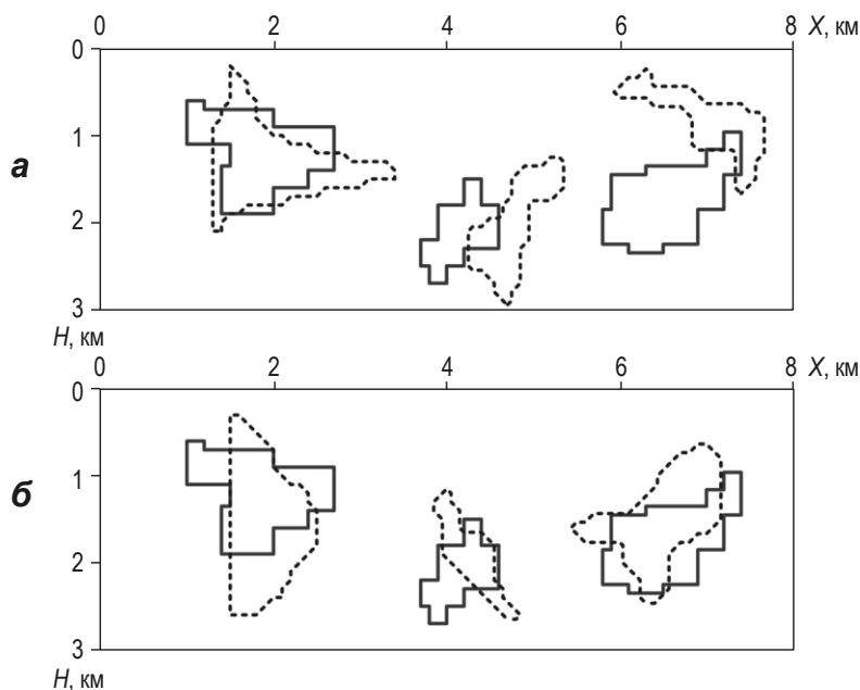
Рис. 5. Решения ОЗГ, отвечающие минимуму невязки полей (а) и максимуму апостериорной вероятности (б). Сплошные линии – источники поля; штриховые – подобранные объекты
